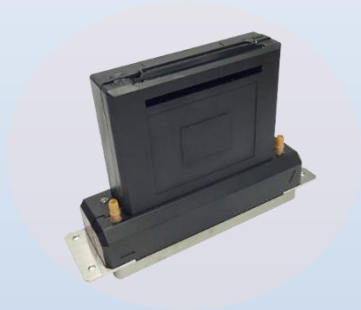
SII1536インクジェットヘッド
